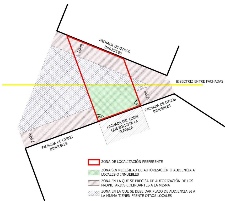
Esquema de zonas de ubicación de terrazas. Caso de fachadas en ángulo
